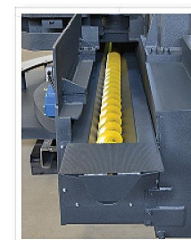
Конвейер для удаления стружки для BMSY360 CGH
