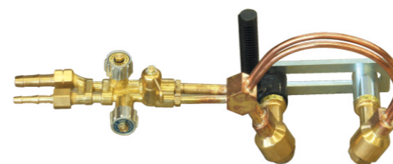
Аксессуары: Двойной резак для подготовки X и V-образных кромок
