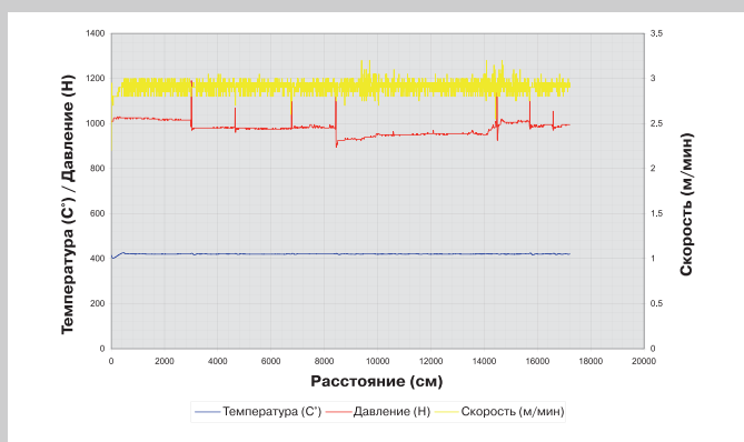
Графическая оценка качества сварного шва (длина: 170 м)
