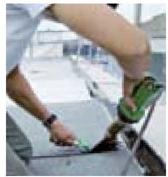
Мощный ELECTRON с широкой щелевой насадкой при сварке битумного покрытия.
